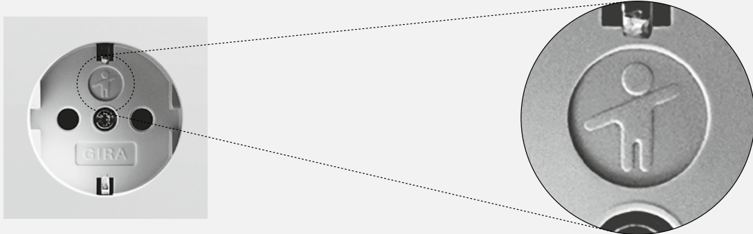
Abbildung: Beispiel für die Abdeckung einer Gira Steckdose mit erhöhtem Berührungsschutz („Kinderschutz“), erkennbar an dem eingepprägten Kinderschutz-Symbol
