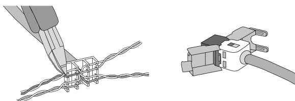
Afbeelding 5: Aansluiting adapterstekker op de Ethernet-leiding
