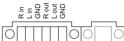
Afbeelding 6: Aansluitbezetting audioverbindingen
