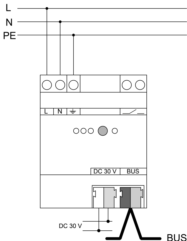
рисунок 3: Пример подключения — сетевое напряжение и линия шины
