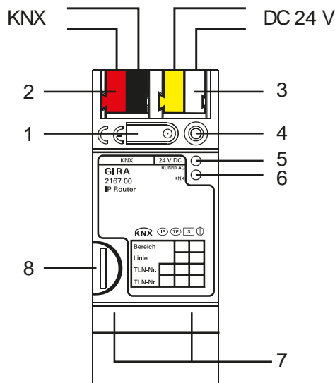
Abbildung 1: KNX IP-Router
