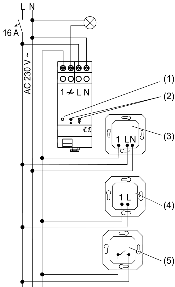
Kuva 1: Liitântäkaavio
