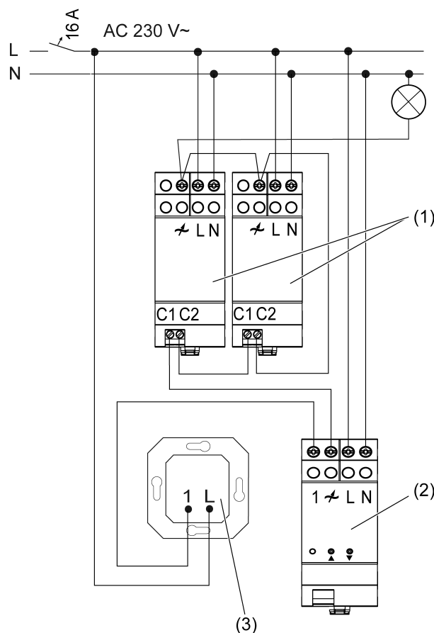
Figura 2: Esempio di collegamento con due elementi di potenza
