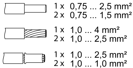
Figure 2: Section transversale de conducteur pouvant être bloquée
