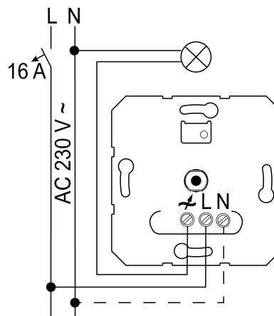
рисунок 3: Монтажная схема
