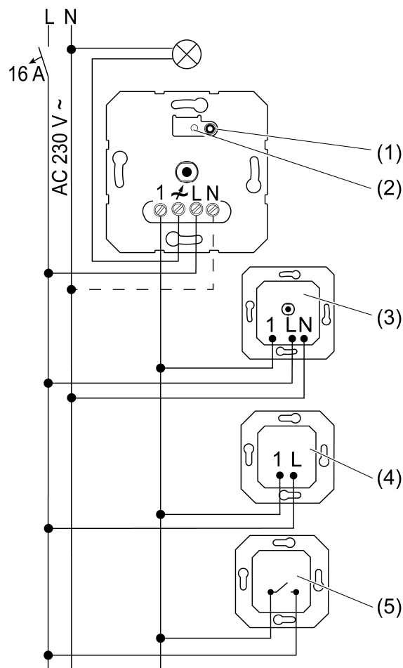
Bilde 3: Koplings skjema med valgfrie biapparater
