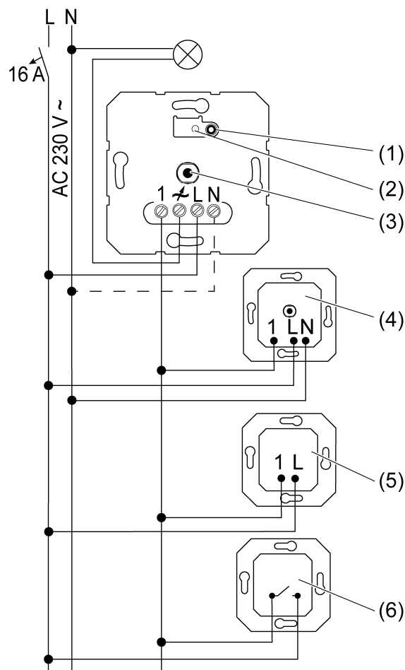
Imagen 3: Plan de conexión con mecanismos auxiliares opcionales
