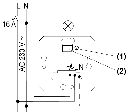
Bilde 1: Koblingskjema
