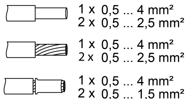
Imagen 2: Secciones de conductor enchufables
