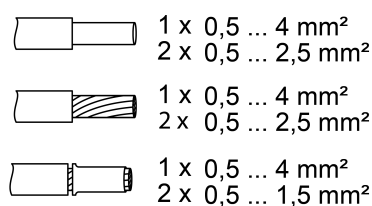
Bild 2: Klemmbare Leiterquerschnitte
