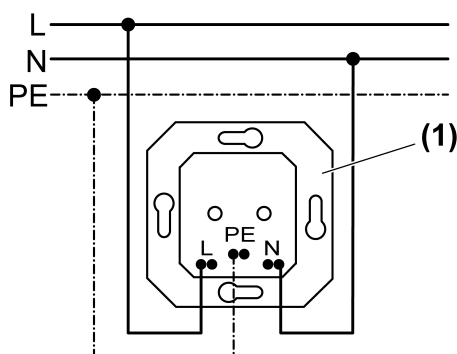
Bild 2: Anschlussplan Einzelsteckdose
