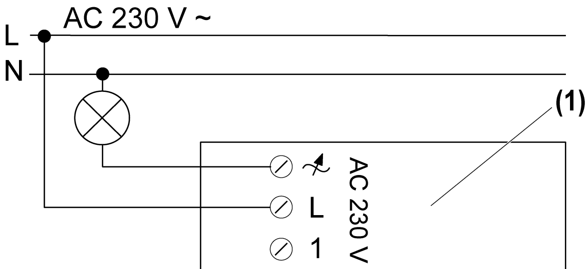
Afbeelding 3: Aansluitschema dimmer
