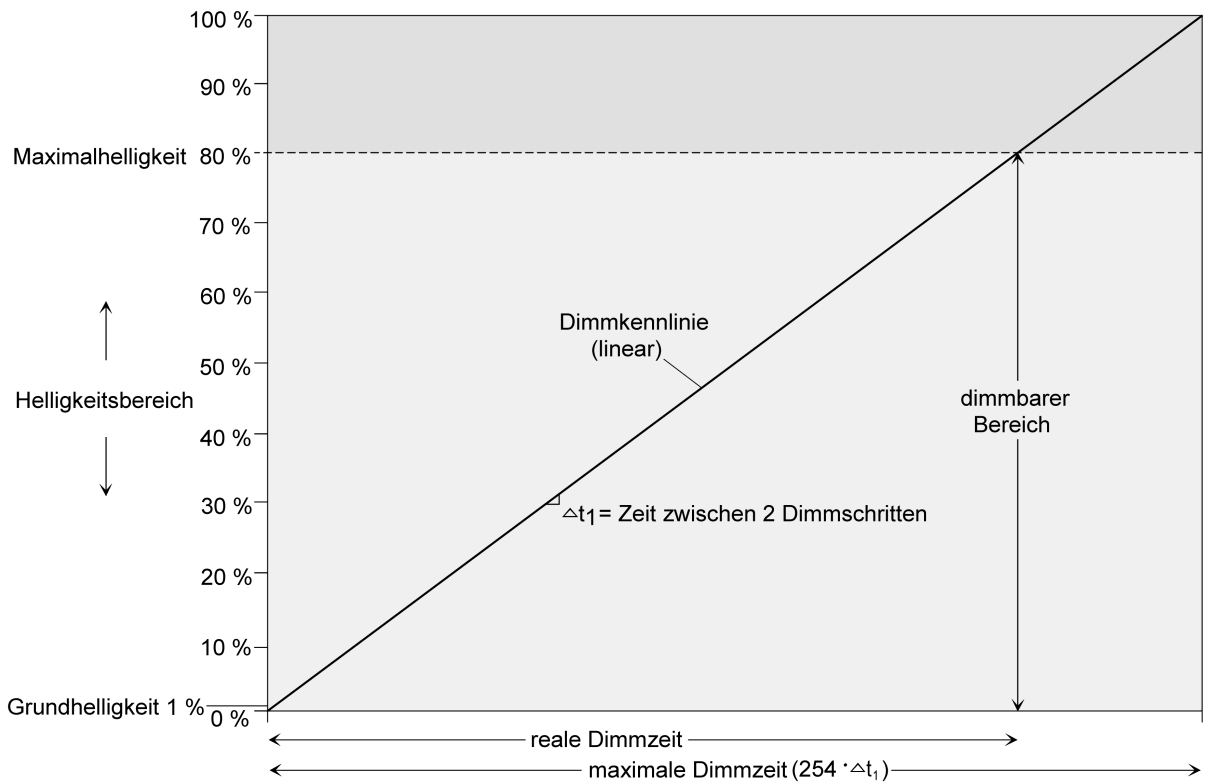
Bild 5: Lineare Dimmkennlinie als Beispiel mit Grundhelligkeit und Maximalhelligkeit
