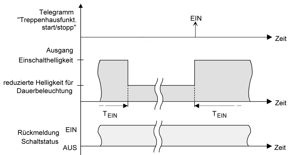
Bild 20: Die Dauerbeleuchtung der Treppenhausfunktion ohne Soft-Funktionen
