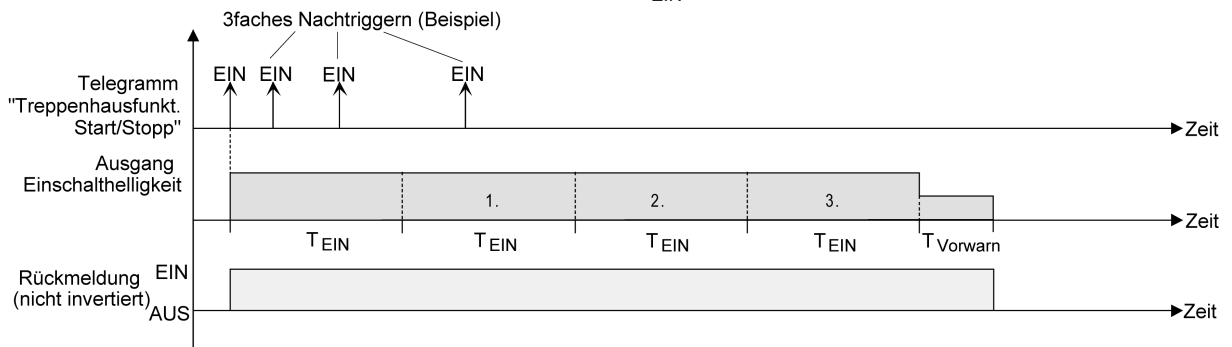
Bild 22: Zeitverlängerung der Treppenhausfunktion
