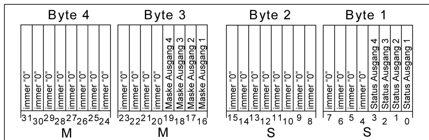
Bild 11: Struktur des Objekts "23" der Sammelrückmeldung für die Ausgänge 1 ... 4
