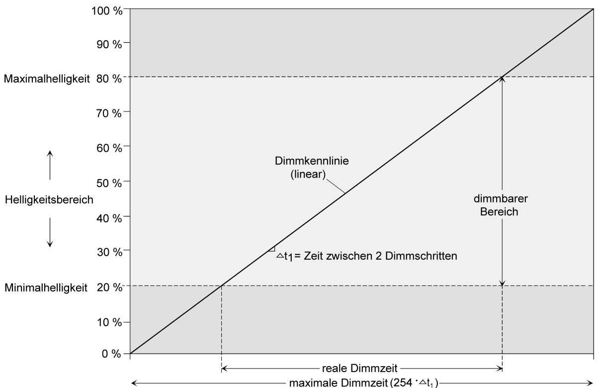
Bild 6: Lineare Dimmkennlinie als Beispiel mit Minimalhelligkeit > 0 % und Maximalhelligkeit
