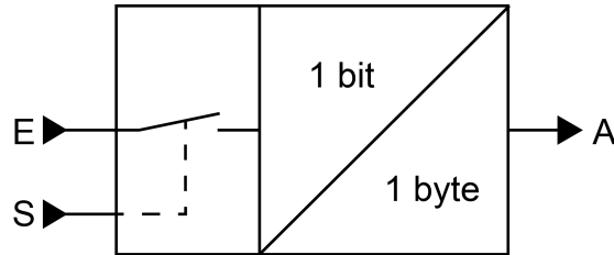
Bild 25: Umsetzer (1 Bit -> 1 Byte)
