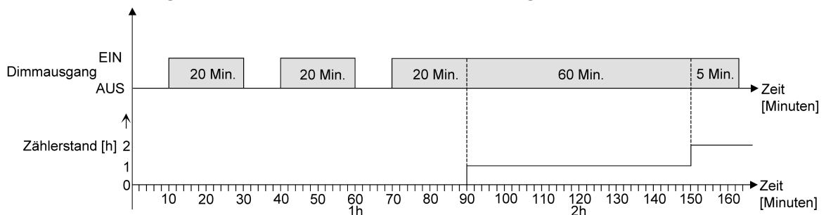
Bild 24: Funktionsweise des Betriebsstundenzählers (am Beispiel gezählter Stunden)
