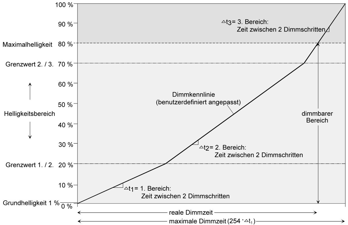
Bild 7: Benutzerdefinierte Dimmkennlinie als Beispiel mit Grundhelligkeit und Maximalhelligkeit
