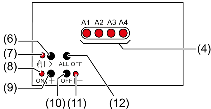
Bild 3: Bedienelemente
