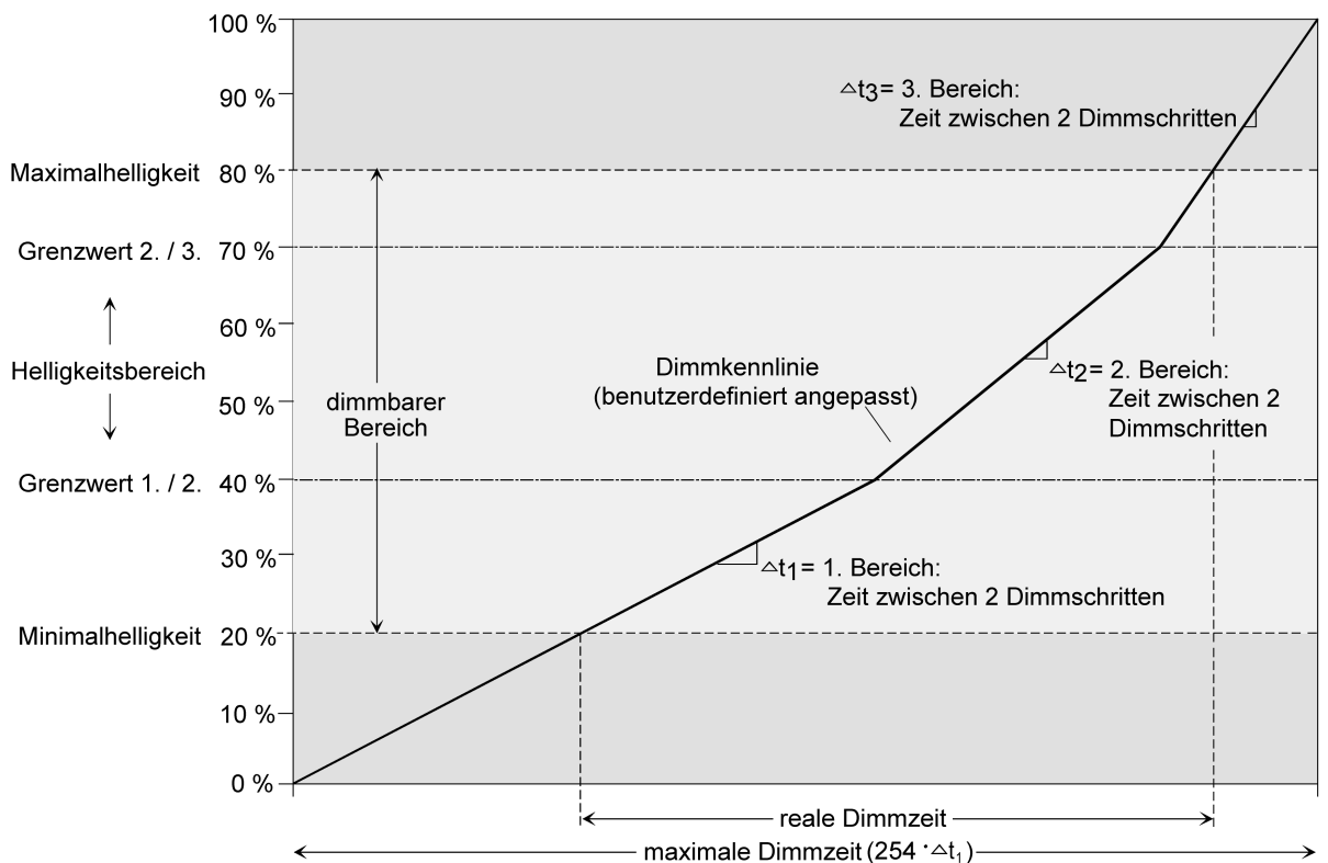
Bild 8: Benutzerdefinierte Dimmkennlinie als Beispiel mit Minimalhelligkeit und
