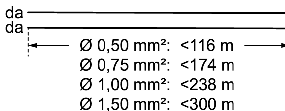
rysunek 4: Długość przewodu DALI
