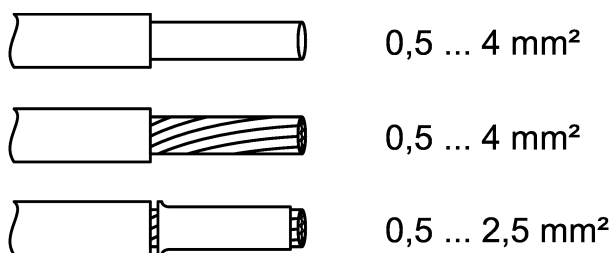
rysunek 5: Zaciskane przekroje przewodów
