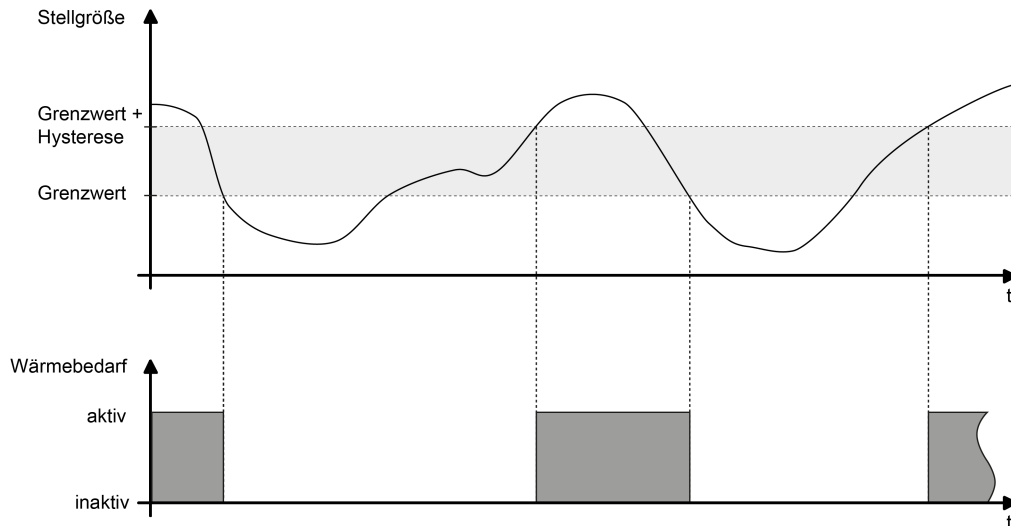
Bild 5: Wärmebedarfsinformation mit beispielhaftem Stellgrößenverlauf
