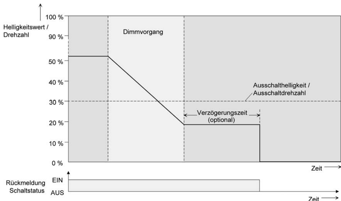
Bild 17: Dimm- und Schaltverhalten der automatischen Ausschaltfunktion
