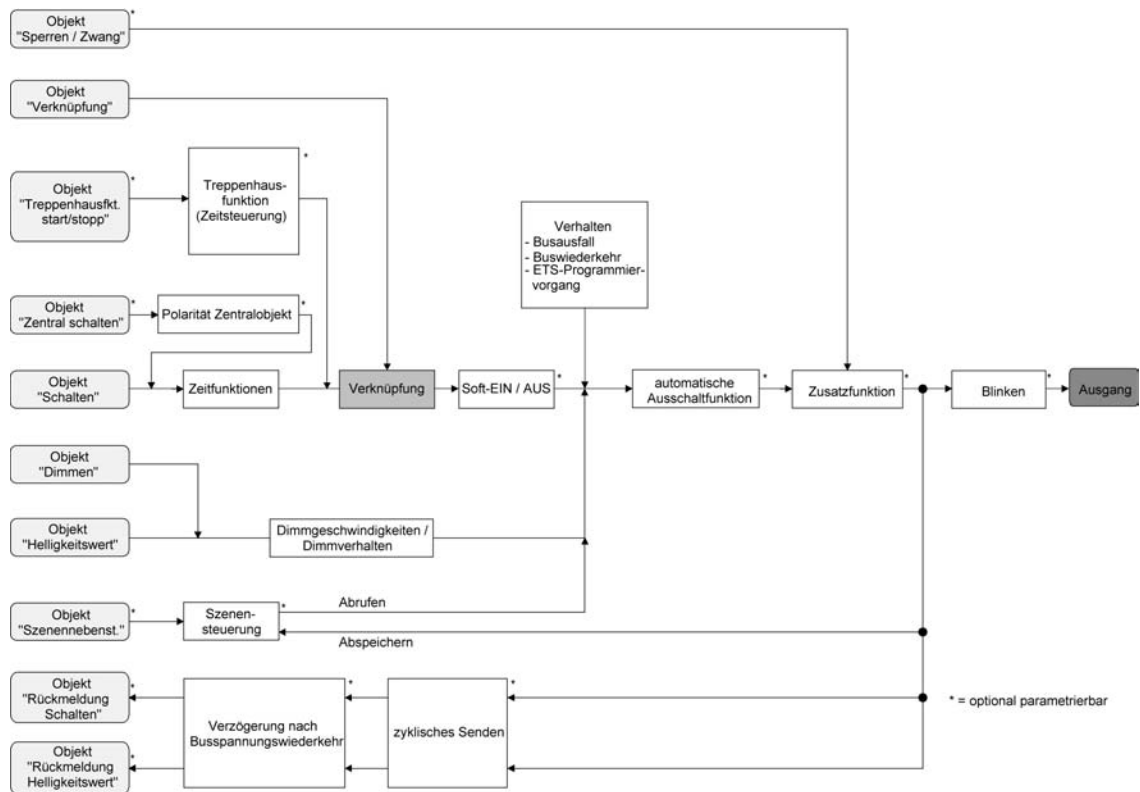
Bild 33: Funktionsschaltbild der Verknüpfungsfunktion
