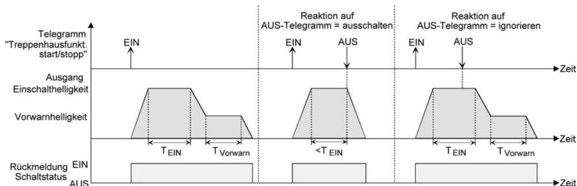
Bild 23: Ausschaltverhalten der Treppenhausfunktion mit Soft-Funktionen (als Beispiel mit Minimalhelligkeit = 0 %)
