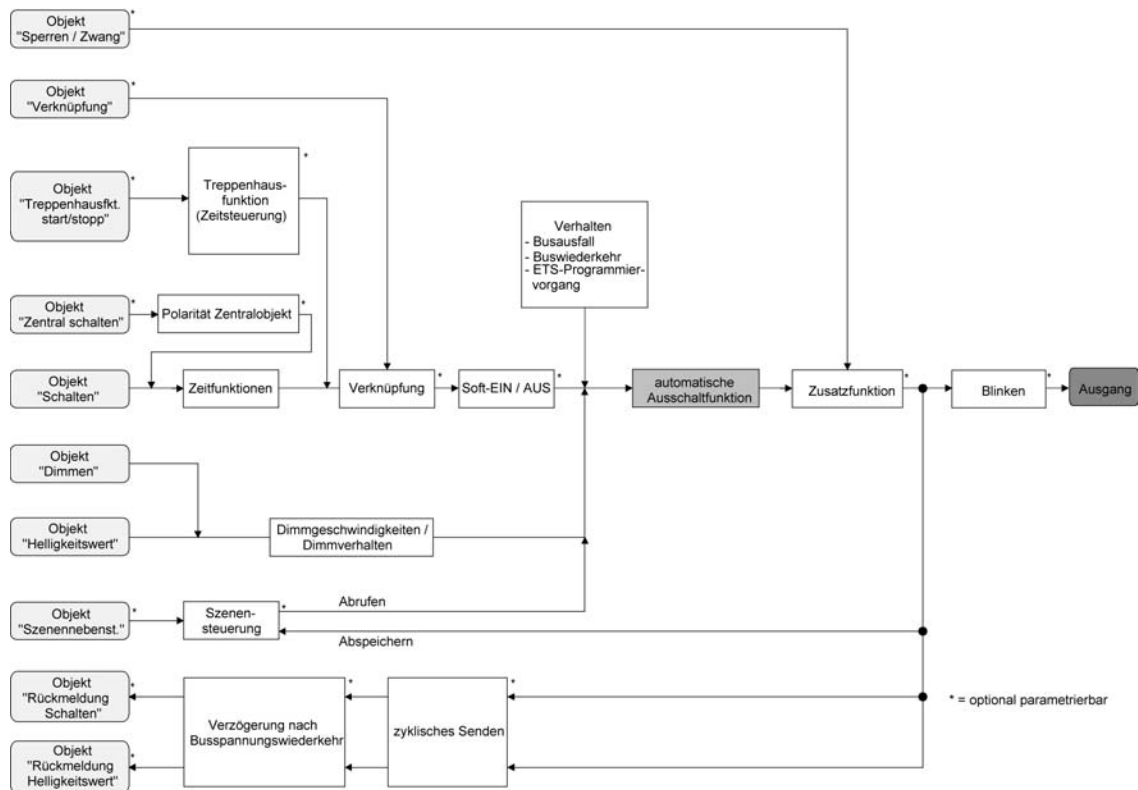
Bild 18: Funktionsschaltbild der automatischen Ausschaltfunktion
