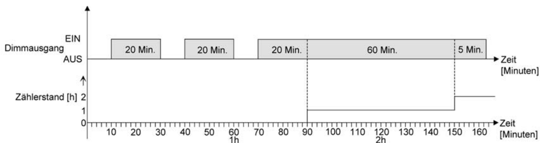
Bild 30: Funktionsweise des Betriebsstundenzählers (am Beispiel eines Vorwärtszählers)
