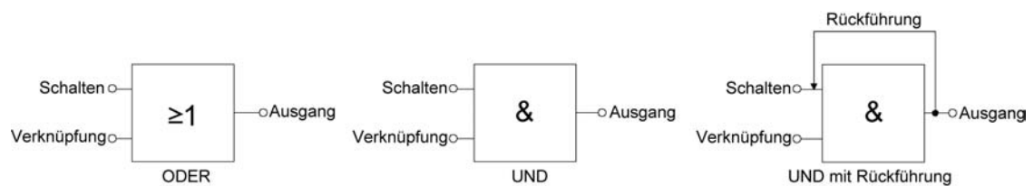
Bild 34: Verknüpfungsarten der Verknüpfungsfunktion
