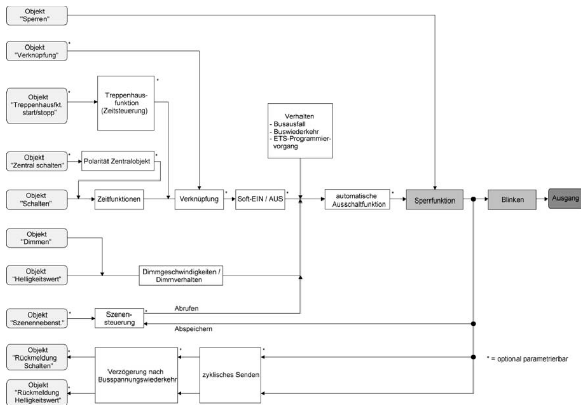
Bild 31: Funktionsschaltbild der Sperrfunktion
