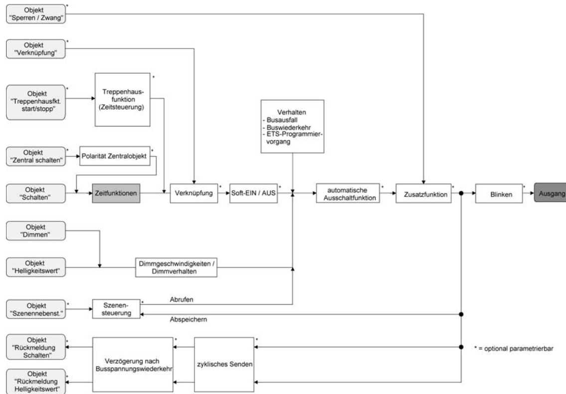
Bild 14: Funktionsschaltbild der Zeitfunktionen
