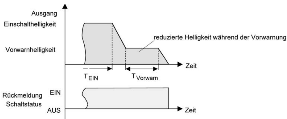
Bild 25: Die Vorwarnfunktion der Treppenhausfunktion mit Soft-AUS-Funktion (als Beispiel mit Minimalhelligkeit = 0 %)
