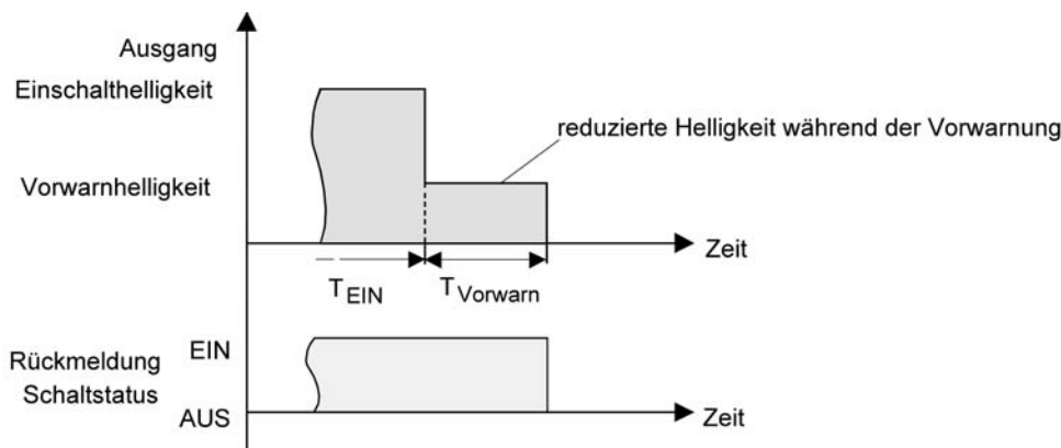
Bild 24: Die Vorwarnfunktion der Treppenhausfunktion ohne Soft-AUS-Funktion
