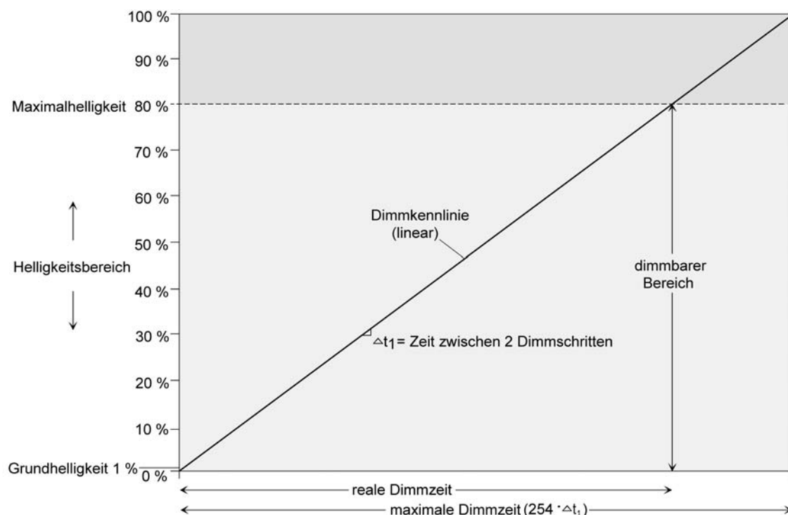
Bild 35: Lineare Dimmkennlinie als Beispiel mit Grundhelligkeit und Maximalhelligkeit
