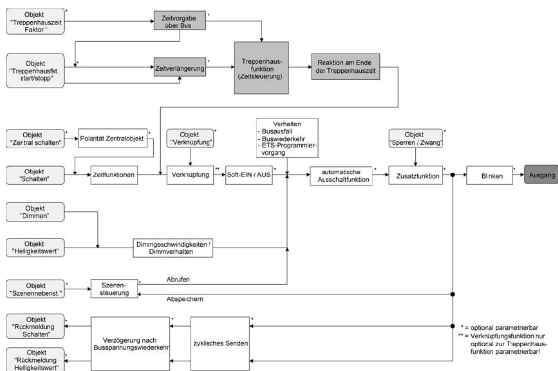
Bild 19: Funktionsschaltbild der Treppenhausfunktion
