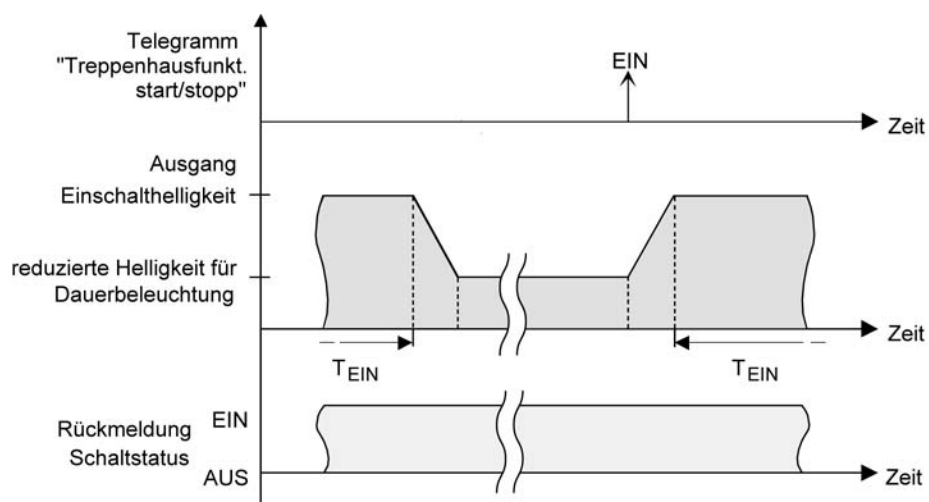
Bild 27: Die Dauerbeleuchtung der Treppenhausfunktion mit Soft-AUS-Funktion
