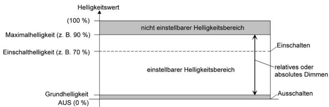
Bild 11: Beispiel eines Helligkeitsbereiches mit Grundhelligkeit
