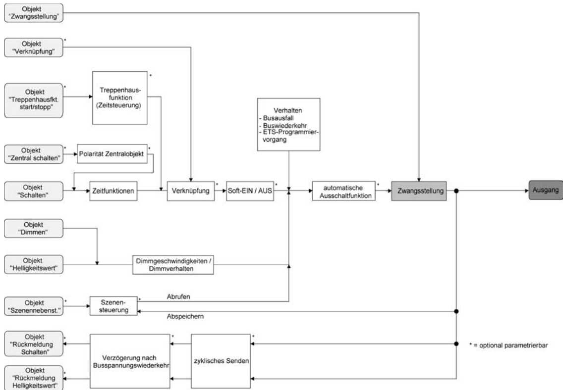
Bild 32: Funktionsschaltbild der Zwangsstellungsfunktion
