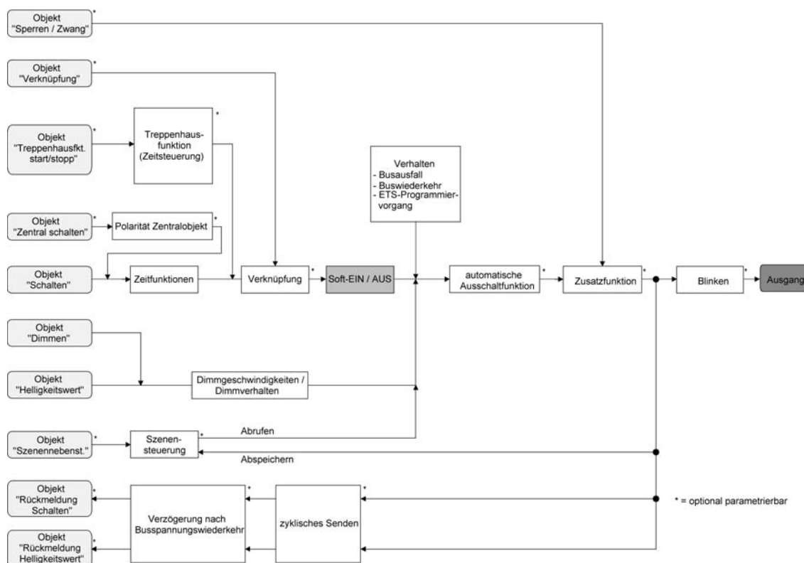
Bild 16: Funktionsschaltbild der Soft-Funktionen
