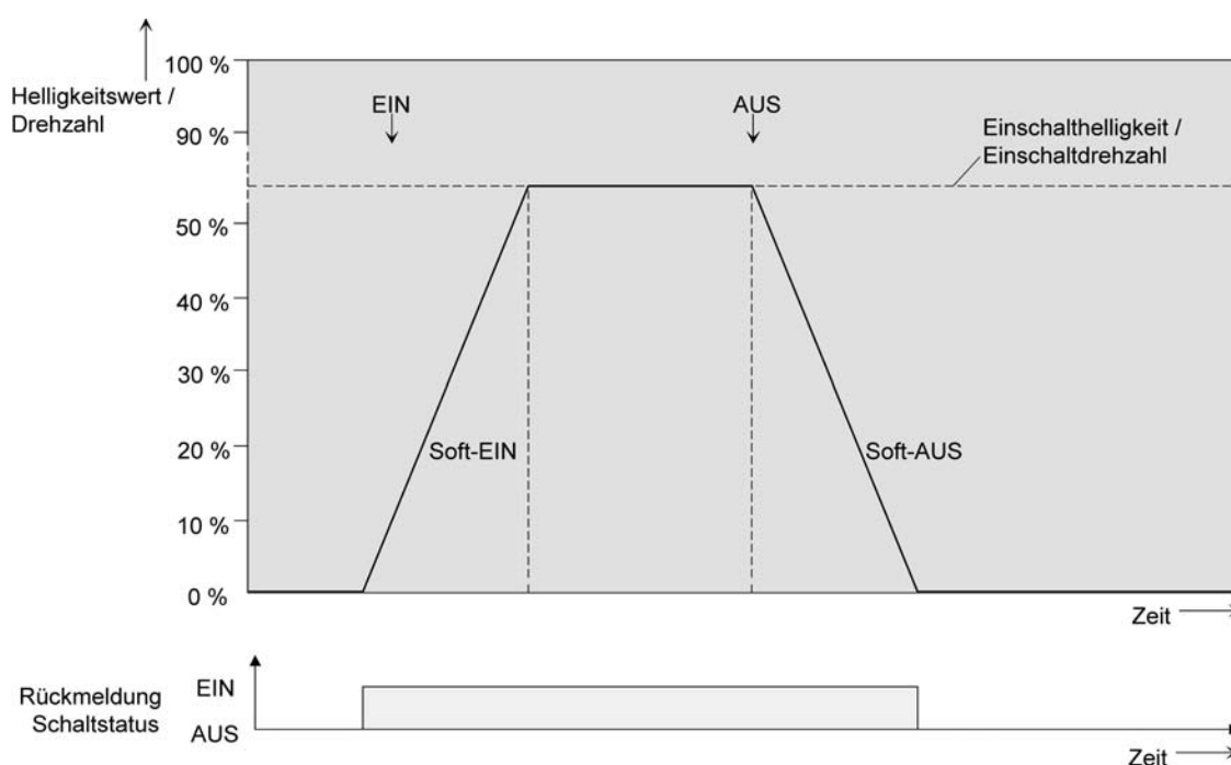
Bild 15: Dimmverhalten der Soft-EIN/AUS-Funktionen (als Beispiel)
