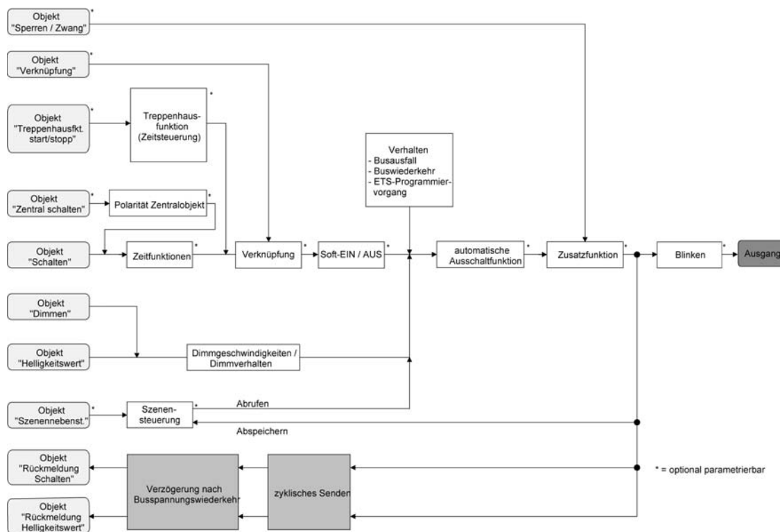
Bild 13: Funktionsschaltbild der Rückmeldungen
