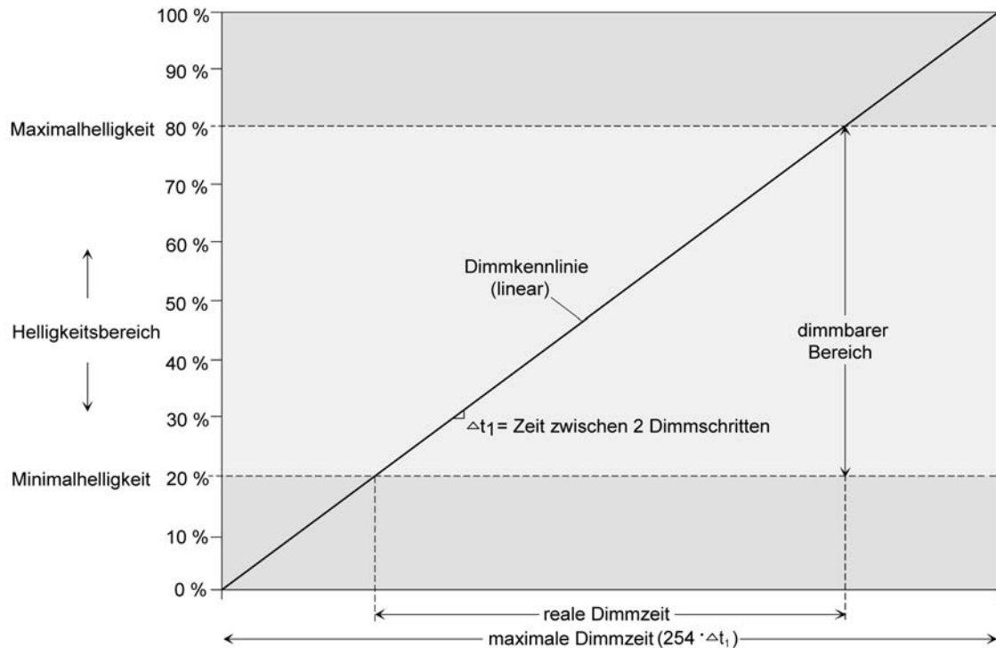
Bild 36: Lineare Dimmkennlinie als Beispiel mit Minimalhelligkeit > 0 % und Maximalhelligkeit
