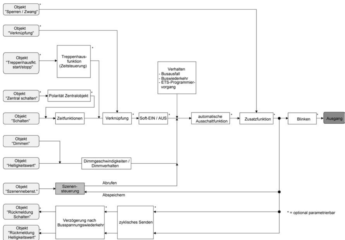
Bild 29: Funktionsschaltbild der Szenenfunktion
