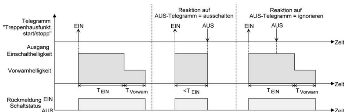
Bild 22: Ausschaltverhalten der Treppenhausfunktion ohne Soft-Funktionen
