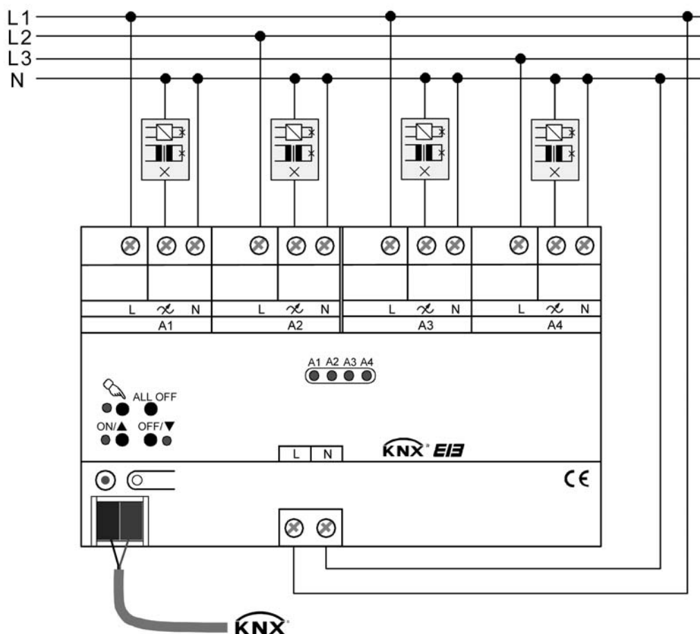
Bild 4: Elektrischer Anschluss (am Beispiel der Gerätevariante 4fach)
