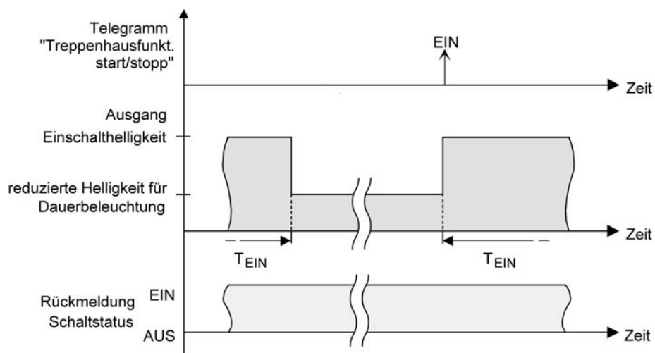
Bild 26: Die Dauerbeleuchtung der Treppenhausfunktion ohne Soft-Funktionen
