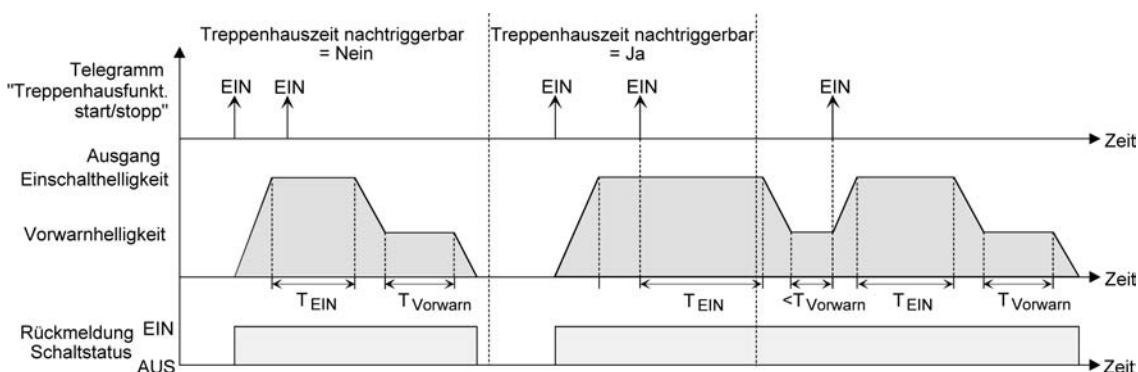
Bild 21: Einschaltverhalten der Treppenhausfunktion mit Soft-Funktionen (als Beispiel mit Minimalhelligkeit = 0 %)
