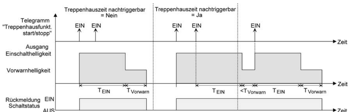
Bild 20: Einschaltverhalten der Treppenhausfunktion ohne Soft-Funktionen
