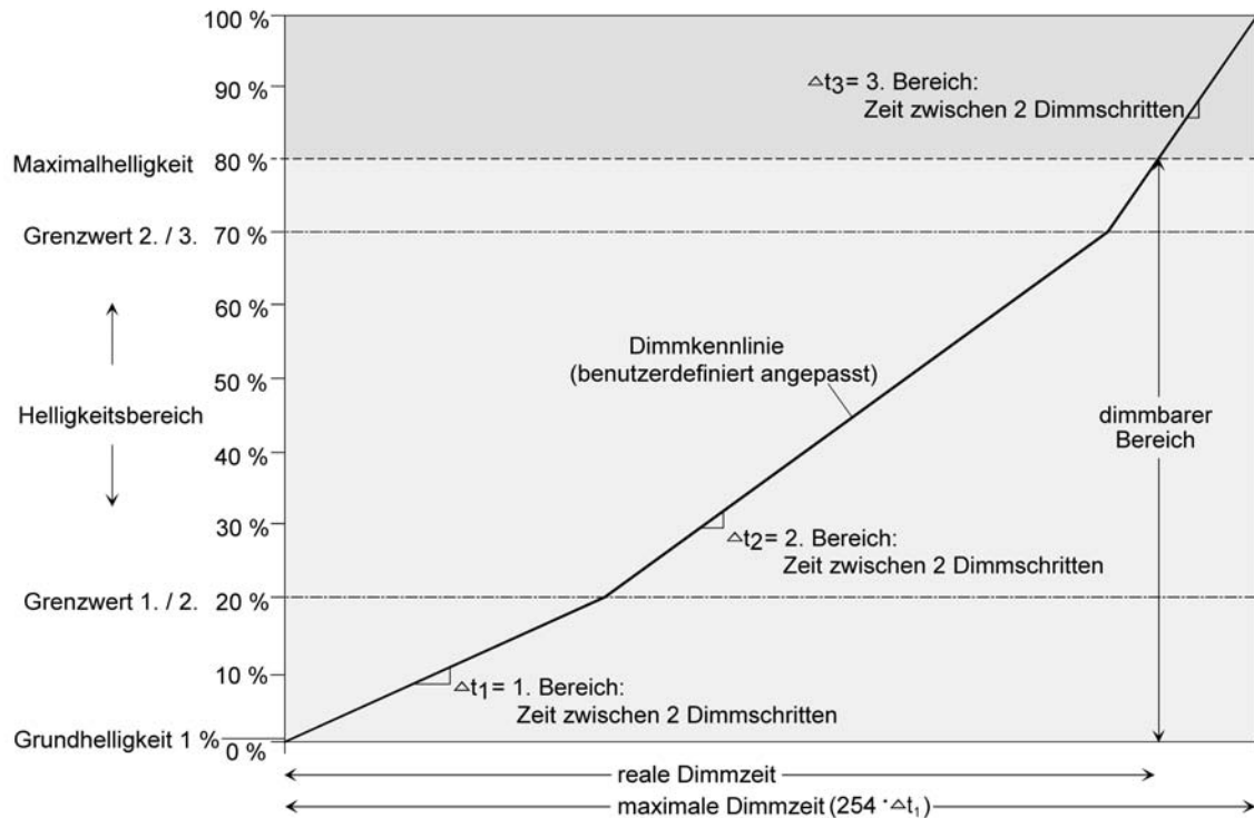
Bild 37: Benutzerdefinierte Dimmkennlinie als Beispiel mit Grundhelligkeit und Maximalhelligkeit
