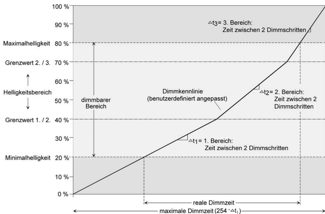
Bild 38: Benutzerdefinierte Dimmkennlinie als Beispiel mit Minimalhelligkeit und Maximalhelligkeit
