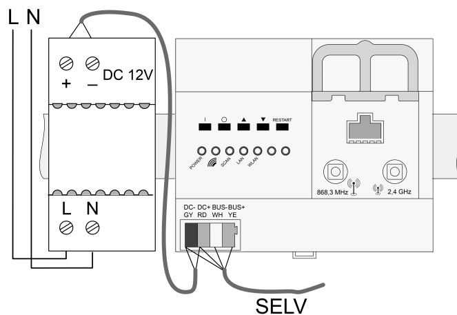
Imagen 3: Plano de conexión
