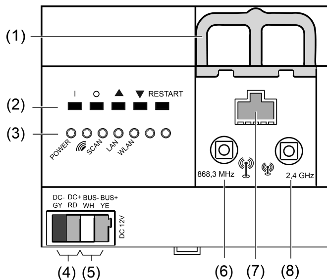
Imagen 1: Vista frontal servidor eNet
