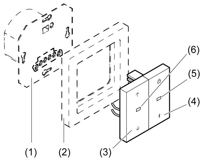
Bild 1: Geräteaufbau
