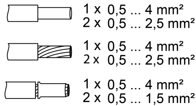
Figura 4: Sección transversal enchufable del conductor
