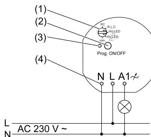
Afbeelding 1: Aansluitschema
