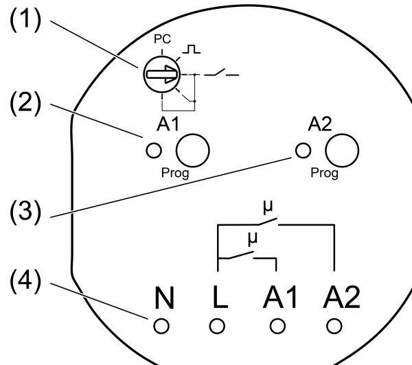
Afbeelding 1: Vooraanzicht
