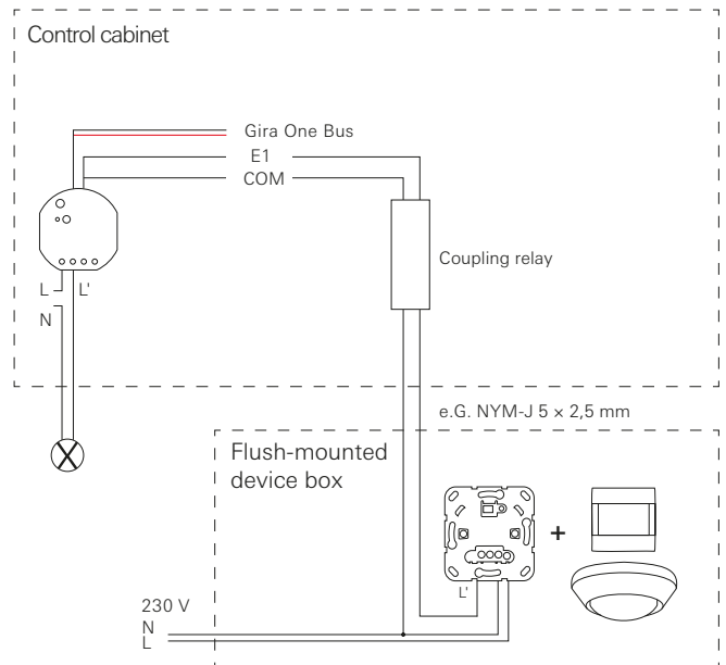
Esempio di connessione
