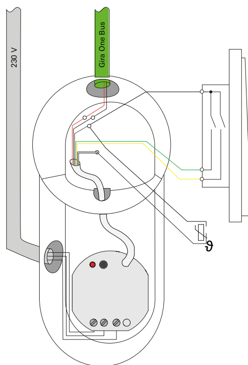
Scatola per dispositivi elettronici con parete divisoria fissa
